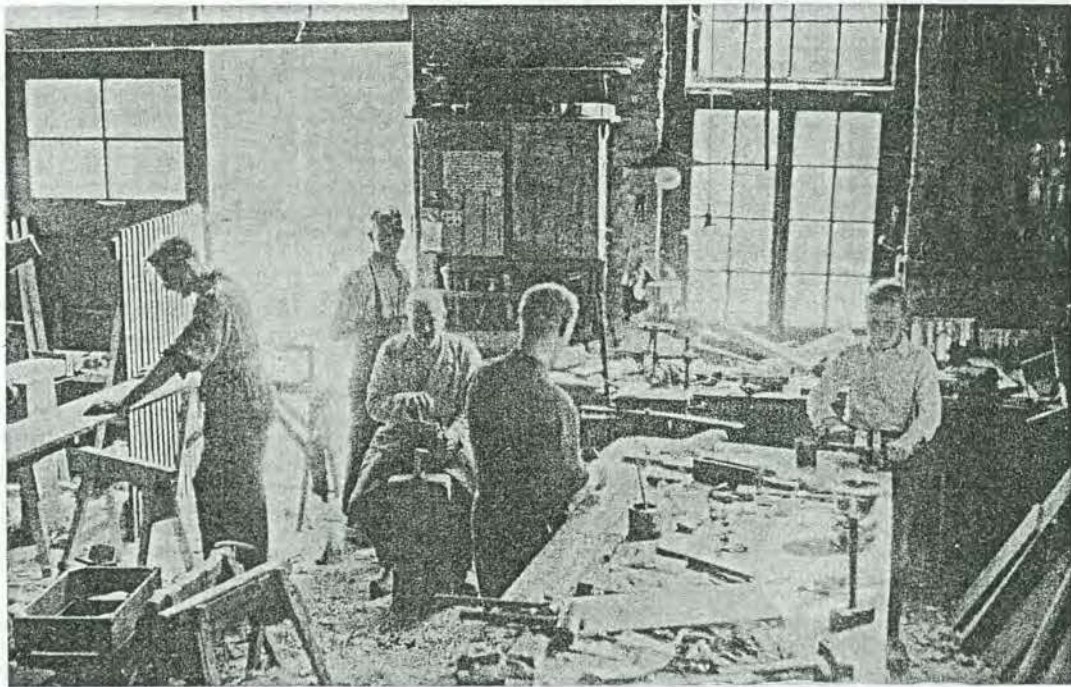
34. De werkplaats van G.H. Diepenhorst in de Pompstraat. Piet van Kekem komt buurten, hij zit op het bankje quasi met een boor in zijn handen, daarnaast staat Freek Diepenhorst. Op de achtergrond is nog een langgatboormachine zichtbaar. In deze timmermanswerkplaats is later de kruiwagenproductie voortgezet die aanvankelijk geschiedde in de schuur tussen bakker Pellikaan (zie 39 het pand links) en het woonhuis van Gerrit Diepenhorst, maar na het overlijden van oom Frêèrik werd dit in de Pompstraat voortgezet door Gerrit en zijn zonen, zijnde Freek en Piet.
